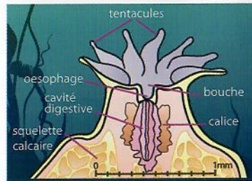
Squelette calcaire
