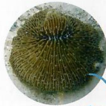
Corail libre
