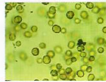
Zooxanthelles
